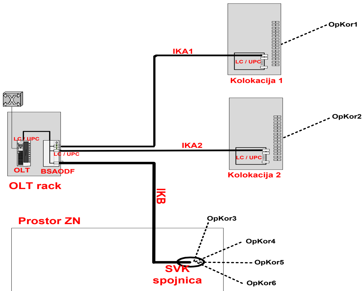
Slika 1. Načini spajanja svjetlovodnog provodnog kabla Operatora korisnika na ODF HT-a
